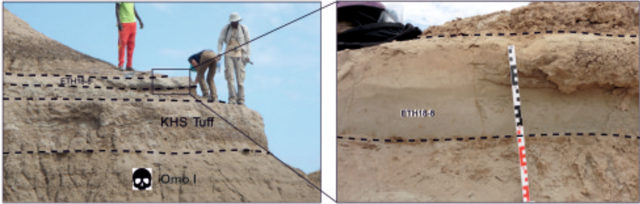
Рис. 2. Положение горизонтов тефры (KHS Tuff и ETH18-8) в разрезе KS (район Омо–Кибिश) (Vidal et al., 2022).
